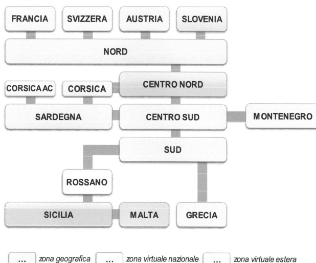
Figura 1 - Topologia di interconnessione delle zone
